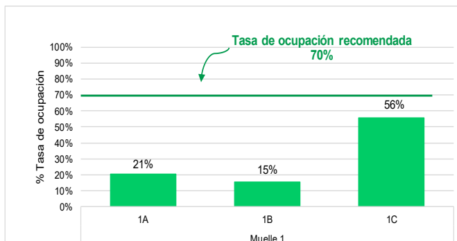
Gráfico N°7 Tasa de ocupación de los muelles del TP General San Martín - TPP Agosto 2021
