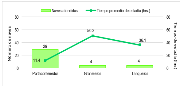
Gráfico N°1 Tiempo promedio de estadía de los amarraderos por tipo de naves en el TP Paíta - TPE, Agosto 2021
