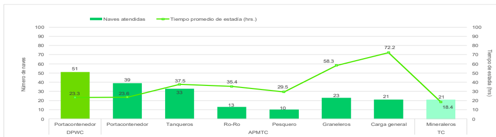
Gráfico N°5 Tiempo promedio de estadía de las naves según tipo, en los amarraderos de los terminales portuarios del Callao administrados por APMTC, DPWC y TC, Agosto 2021
