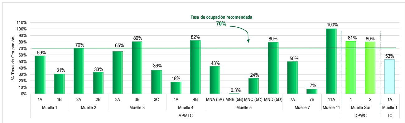
Gráfico N°10 Tasa de ocupación de los muelles de los terminales portuarios del Callao administrados por APMTC, DPWC y TCSA, Agosto 2021
