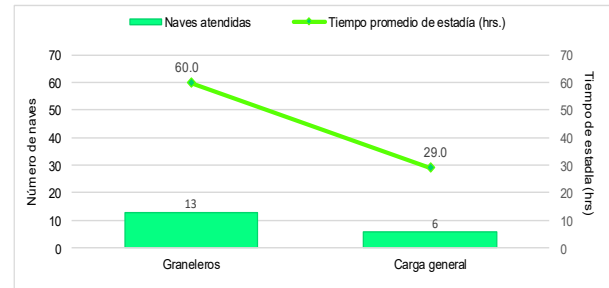
Gráfico N°4 Tiempo promedio de estadía de los amarraderos por tipo de nave en el TP Salaverry Terminal Internacional - STI, Agosto 2021
