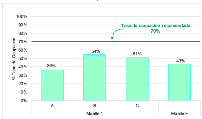
Gráfico N°8 Tasa de ocupación de los muelles de TP Matarani - TISUR Agosto 2021
