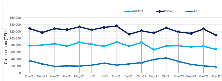
Gráfico N°1 Movimiento de contenedores en los terminales portuarios del Callao y Paita que emplearon grúas pórtico, enero 2021 a abril 2022
