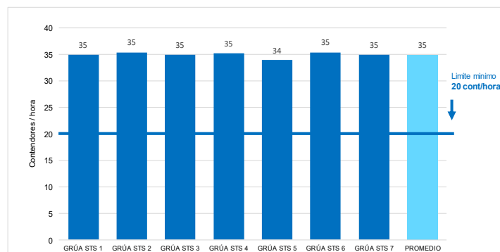
Gráfico N°4 Productividad de grúas pórtico en el terminal Muelle Sur - DPWC, abril 2022
