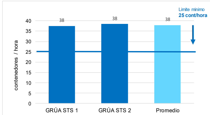
Gráfico N°5 Productividad de grúas pórtico en el Terminal Portuario de Paita - TPE, Abril 2022
