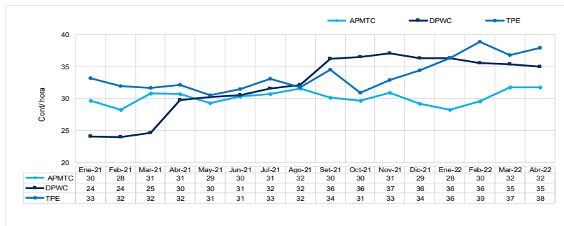
Gráfico N°2 Productividad de grúas pórtico en los terminales portuarios del Callao y Paita, enero 2021 a abril 2022
