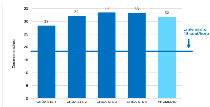
Gráfico N°3 Productividad de grúas pórtico en el TNM Callao - APMTC, abril 2022
