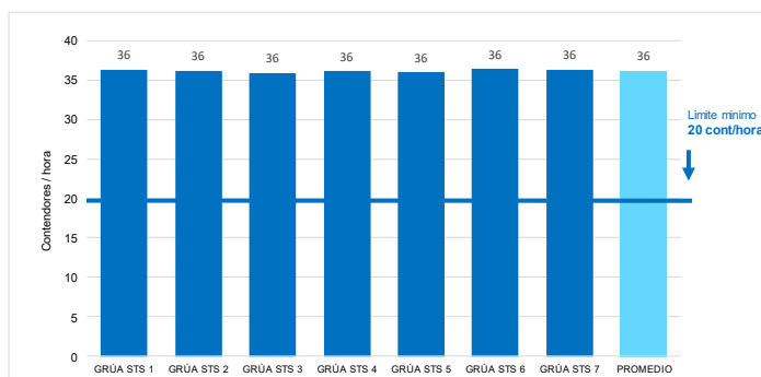
Gráfico N°4 Productividad de grúas pórtico en el terminal Muelle Sur - DPWC, año 2022
