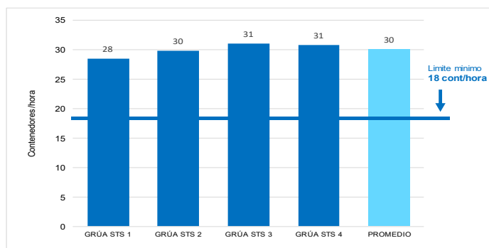
Gráfico N°3 Productividad de grúas pórtico en el TNM Callao - APMTC, año 2022
