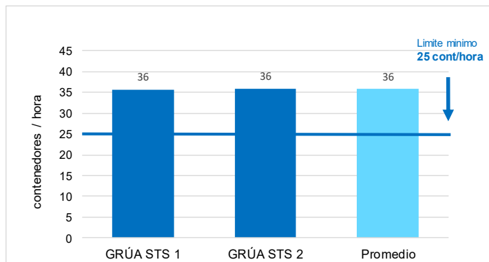
Gráfico N°5 Productividad de grúas pórtico en el Terminal Portuario de Paita - TPE, año 2022
