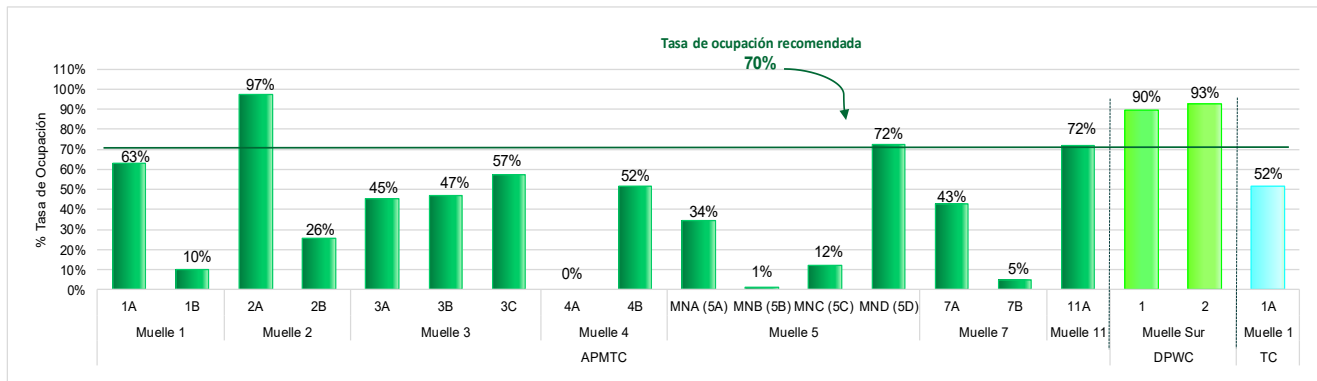
Gráfico N°10 Tasa de ocupación de los muelles de los terminales portuarios del Callao administrados por APMTC, DPWC y TCSA, Enero 2021
