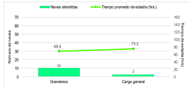
Gráfico N°4 Tiempo promedio de estadía de los amarraderos por tipo de nave en el TP Salaverry Terminal Internacional - STI, Enero 2021
