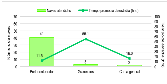
Gráfico N°1 Tiempo promedio de estadía de los amarraderos por tipo de naves en el TP Paíta - TPE, Enero 2021
