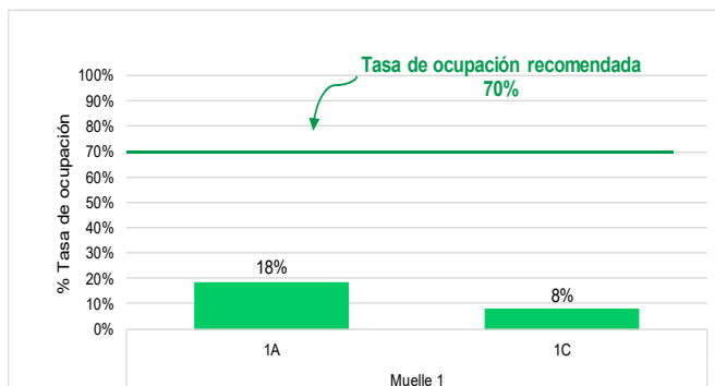
Gráfico N°7 Tasa de ocupación de los muelles del TP General San Martín - TPP Enero 2021
