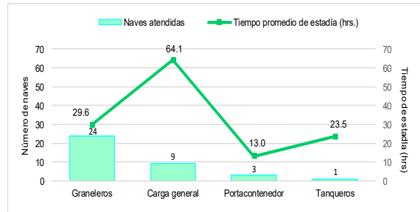
Gráfico N°2 Número de naves atendidas y tiempo de estadía de los amarraderos de TP Matarani - TISUR, Enero 2021
