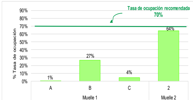
Gráfico N°6 Tasa de ocupación de los amarraderos de TP Paita -TPE Enero 2021
