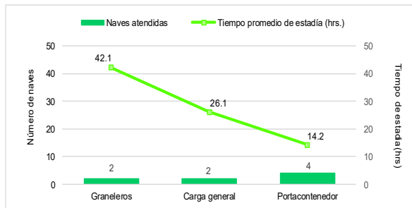
Gráfico N°3 Tiempo promedio de estadía de los amarraderos por tipo de nave en el TP General San Martín - TPP, Enero 2021
