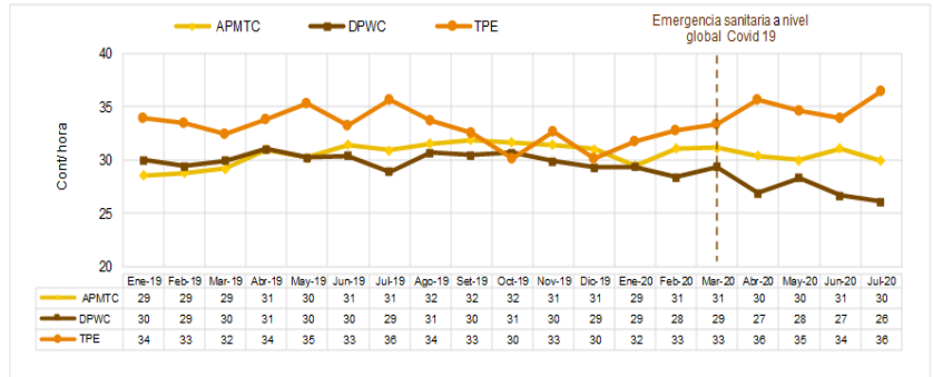
Gráfico N°2 Productividad de grúas pórtico en los terminales portuarios del Callao y Paita, enero 2019 a julio 2020
