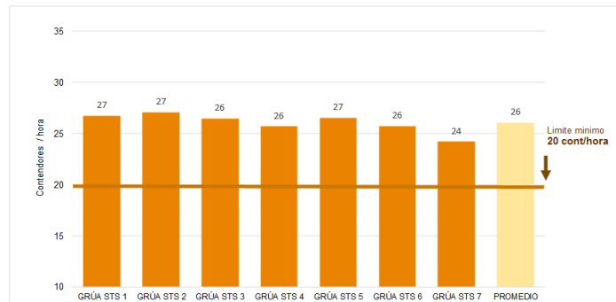
Gráfico N°4 Productividad de grúas pórtico en el terminal Muelle Sur - DPWC, julio 2020
