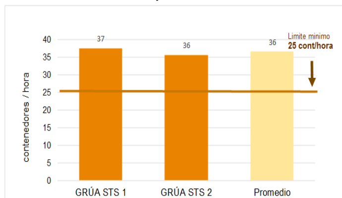
Gráfico N°5 Productividad de grúas pórtico en el Terminal Portuario de Paita - TPE, julio 2020
