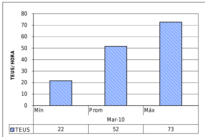
1.6. PERÚ: MOVIMIENTO DE TEUS / HORA EN NAVES GEARLESS UTILIZANDO DOS GRÚAS PÓRTICO, MES DE MARZO 2010. (*)
