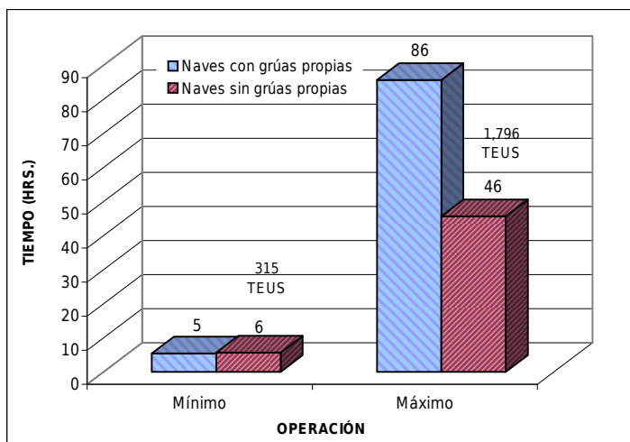
1.4. PERÚ: TIEMPO DE OPERACIÓN DE NAVES PORTACONTENEDORES, MES DE MARZO 2010.
