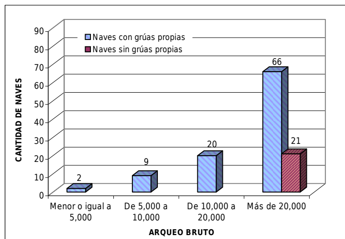
1.3. PERÚ: NAVES PORTACONTENEDORES POR ARQUEO BRUTO, MES DE MARZO 2010.
