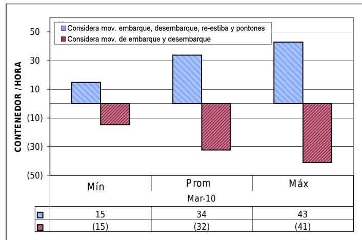
1.5. PERÚ: MOVIMIENTO DE CONTENEDORES / HORA EN NAVES GEARLESS UTILIZANDO DOS GRÚAS PÓRTICO, MES DE MARZO 2010. (*)
