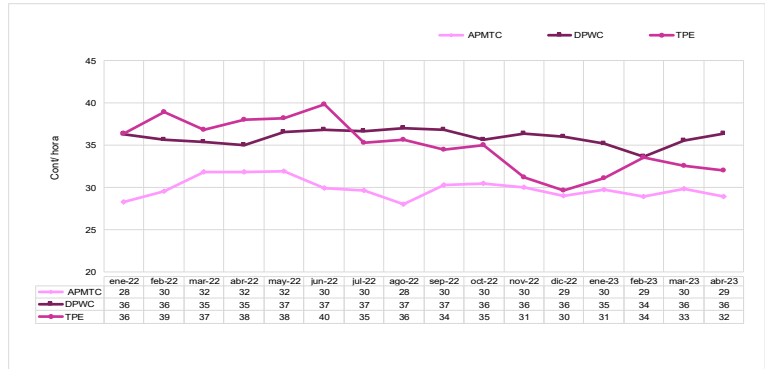
Gráfico N°2 Productividad de grúas pórtico en los terminales portuarios del Callao y Paita, enero 2022 a abril 2023
