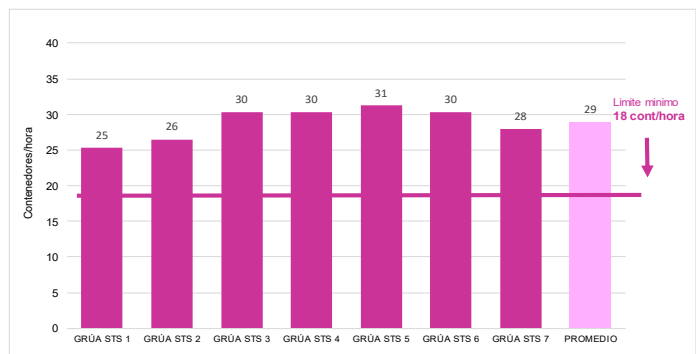
Gráfico N°3 Productividad de grúas pórtico en el TNM Callao - APMTC, abril 2023
