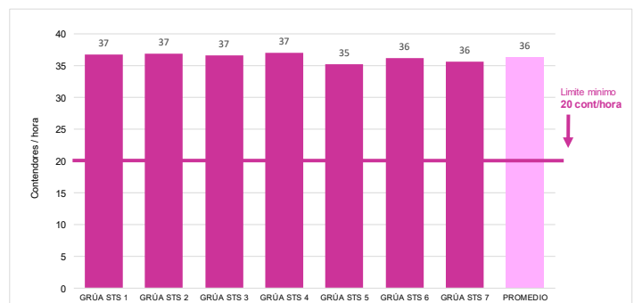
Gráfico N°4 Productividad de grúas pórtico en el terminal Muelle Sur - DPWC, abril 2023
