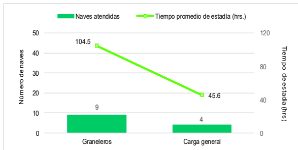
Gráfico N°3 Tiempo promedio de estadía de los amarraderos por tipo de nave en el TP General San Martín - TPP, Mayo 2021
