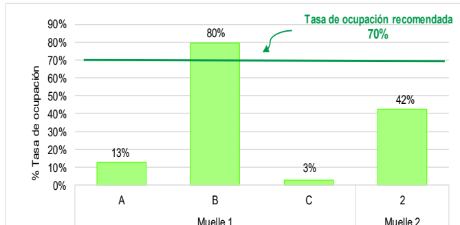
Gráfico N°6 Tasa de ocupación de los amarraderos de TP Paíta -TPE Mayo 2021
