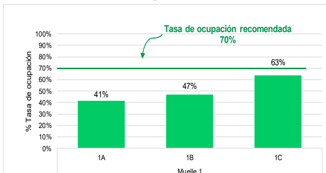
Gráfico N°7 Tasa de ocupación de los muelles del TP General San Martín - TPP Mayo 2021
