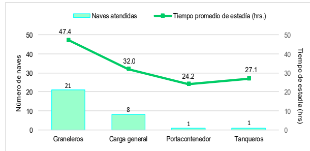
Gráfico N°2 Número de naves atendidas y tiempo de estadía de los amarraderos de TP Matarani - TISUR, Mayo 2021
