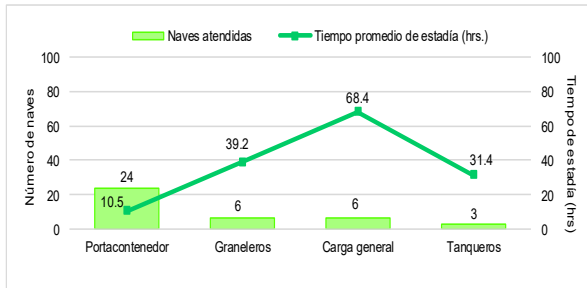
Gráfico N°1 Tiempo promedio de estadía de los amarraderos por tipo de naves en el TP Paíta - TPE, Mayo 2021
