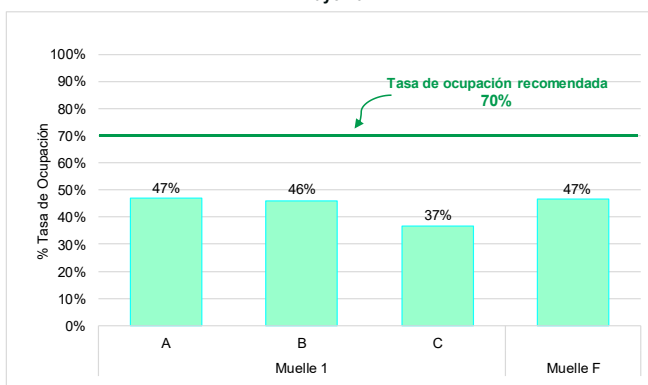
Gráfico N°8 Tasa de ocupación de los muelles de TP Matarani - TISUR Mayo 2021
