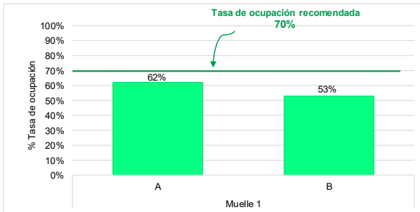
Gráfico N°9 Tasa de ocupación de los muelles de TP Salaverry - STI Mayo 2021
