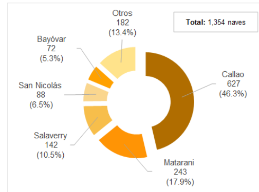
Gráfico N° 5 Naves graneleros recibidas según puerto año 2020
