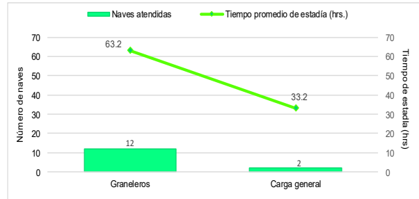
Gráfico N°4 Tiempo promedio de estadía de los amarraderos por tipo de nave en el TP Salaverry Terminal Internacional - STI, Setiembre 2021
