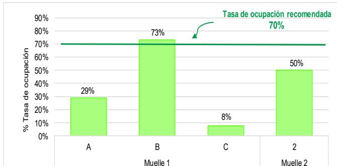
Gráfico N°6 Tasa de ocupación de los amarraderos de TP Paita -TPE Setiembre 2021
