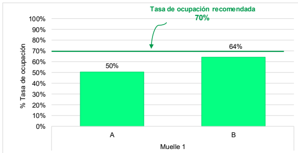
Gráfico N°9 Tasa de ocupación de los muelles de TP Salaverry - STI Setiembre 2021
