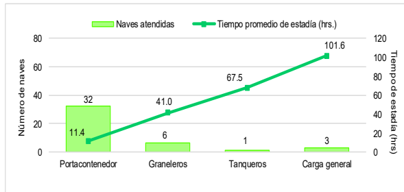
Gráfico N°1 Tiempo promedio de estadía de los amarraderos por tipo de naves en el TP Paíta - TPE, Setiembre 2021
