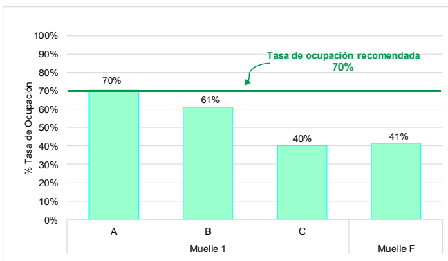
Gráfico N°8 Tasa de ocupación de los muelles de TP Matarani - TISUR Setiembre 2021
