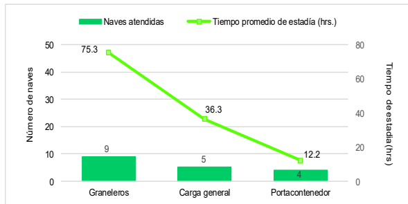
Gráfico N°3 Tiempo promedio de estadía de los amarraderos por tipo de nave en el TP General San Martín - TPP, Setiembre 2021
