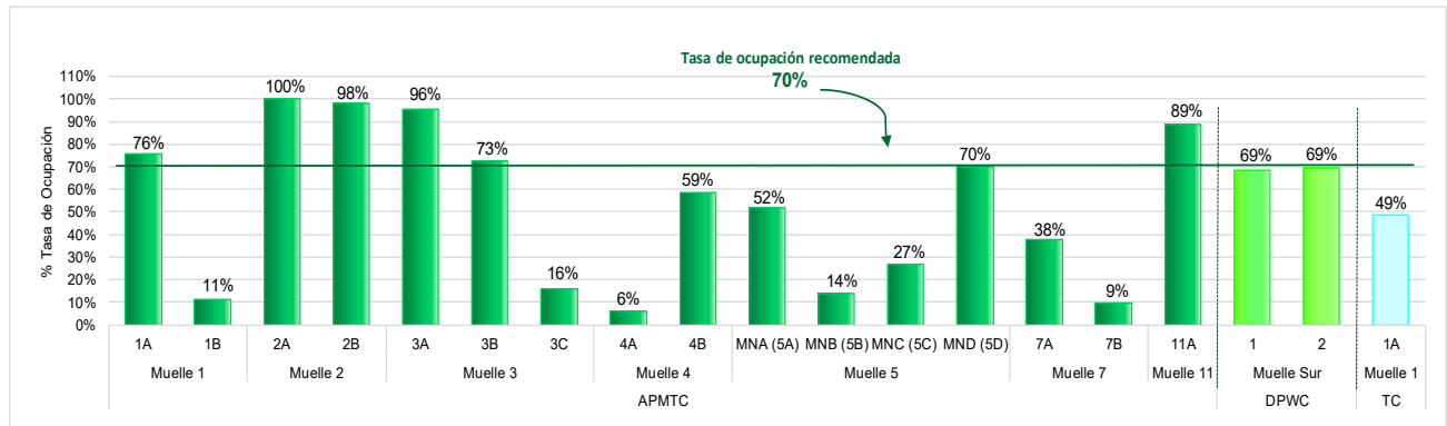
Gráfico N°10 Tasa de ocupación de los muelles de los terminales portuarios del Callao administrados por APMTC, DPWC y TCSA, Setiembre 2021
