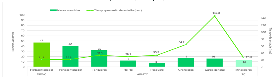
Gráfico N°5 Tiempo promedio de estadía de las naves según tipo, en los amarraderos de los terminales portuarios del Callao administrados por APMTC, DPWC y TC, Setiembre 2021
