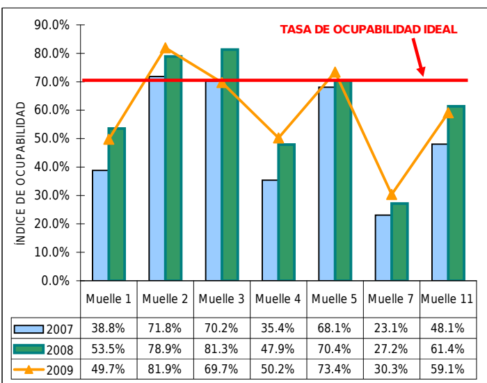
GRÁFICO 1.4 ÍNDICE DE OCUPABILIDAD EN LOS MUELLES DEL TPC, AÑO 2007 - 09.
