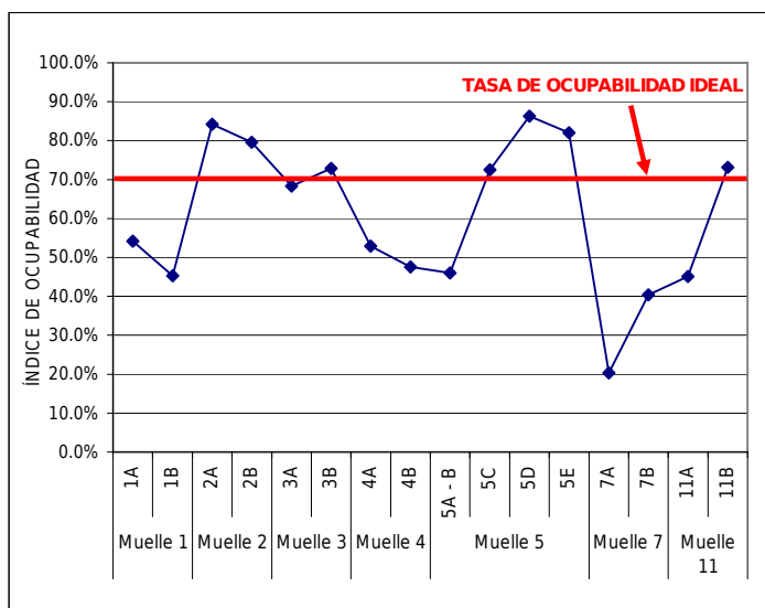
GRÁFICO 1.5 ÍNDICE DE OCUPABILIDAD EN LOS AMARRADEROS DEL TPC, AÑO 2009.
