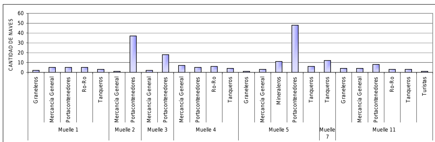
GRÁFICO 1.3 TIPO DE NAVES RECIBIDAS POR MUELLE EN EL TPC, FEBRERO 2010.
