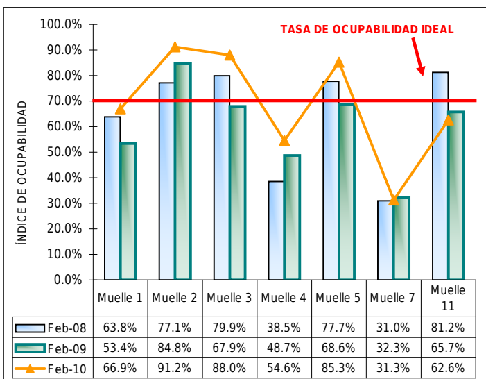
GRÁFICO 1.4 ÍNDICE DE OCUPABILIDAD EN LOS MUELLES DEL TPC, FEBRERO 2008 - 10.
