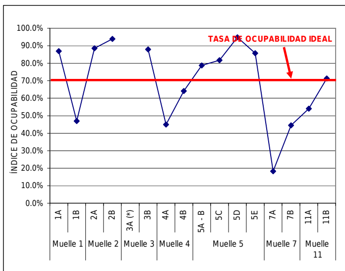
GRÁFICO 1.5 OCUPABILIDAD EN LOS AMARRADEROS DEL TPC, FEBRERO 2010.
