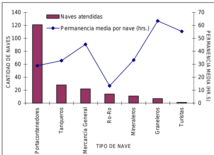
GRÁFICO 1.2 PERMANENCIA DE LAS NAVES RECIBIDAS EN EL TPC, FEBRERO 2010.
