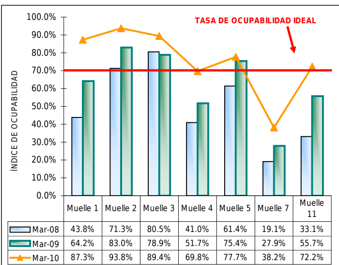
GRÁFICO 1.4 ÍNDICE DE OCUPABILIDAD EN LOS MUELLES DEL TPC, MARZO 2008 - 10.
