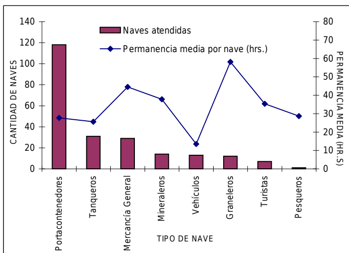
GRÁFICO 1.2 PERMANENCIA DE LAS NAVES RECIBIDAS EN EL TPC, MARZO 2010.
