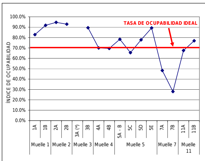
GRÁFICO 1.5 OCUPABILIDAD EN LOS AMARRADEROS DEL TPC, MARZO 2010.
