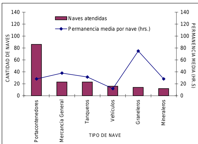
GRÁFICO 1.2 PERMANENCIA DE LAS NAVES RECIBIDAS EN EL TPC, MAYO 2010.
