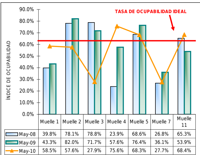
GRÁFICO 1.4 ÍNDICE DE OCUPABILIDAD EN LOS MUELLES DEL TPC, MAYO 2008 - 10.
