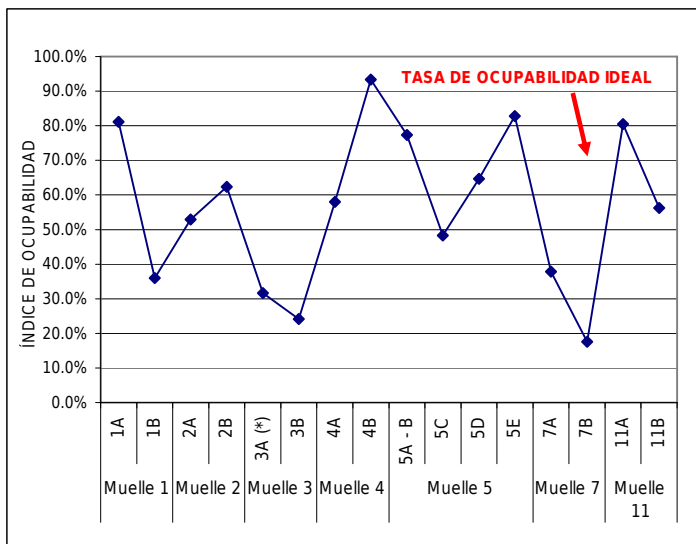
GRÁFICO 1.5 OCUPABILIDAD EN LOS AMARRADEROS DEL TPC, MAYO 2010.
