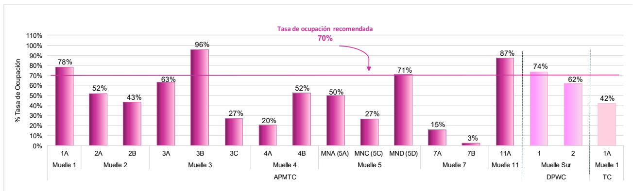
Gráfico N°10 Tasa de ocupación de los muelles de los terminales portuarios del Callao administrados por APMTC, DPWC y TCSA, Enero 2023
