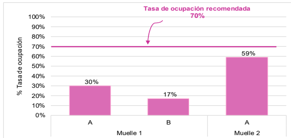
Gráfico N°9 Tasa de ocupación de los muelles de TP Salaverry - STI Enero 2023
