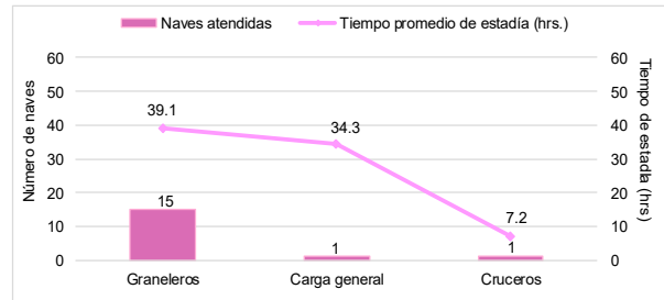
Gráfico N°4 Tiempo promedio de estadía de los amarraderos por tipo de nave en el TP Salaverry Terminal Internacional - STI, Enero 2023
