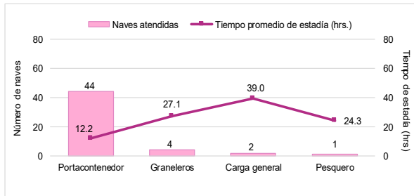
Gráfico N°1 Tiempo promedio de estadía de los amarraderos por tipo de naves en el TP Paita - TPE, Enero 2023
