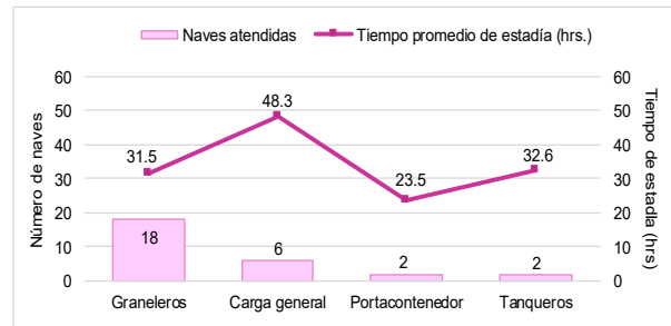
Gráfico N°2 Número de naves atendidas y tiempo de estadía de los amarraderos de TP Matarani - TISUR, Enero 2023
