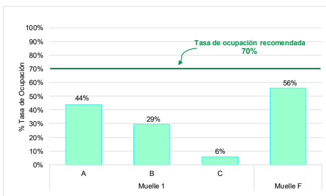
Gráfico N°8 Tasa de ocupación de los muelles de TP Matarani - TISUR Julio 2021
