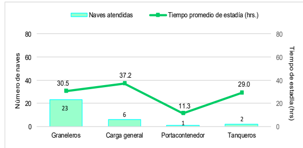
Gráfico N°2 Número de naves atendidas y tiempo de estadía de los amarraderos de TP Matarani - TISUR, Julio 2021
