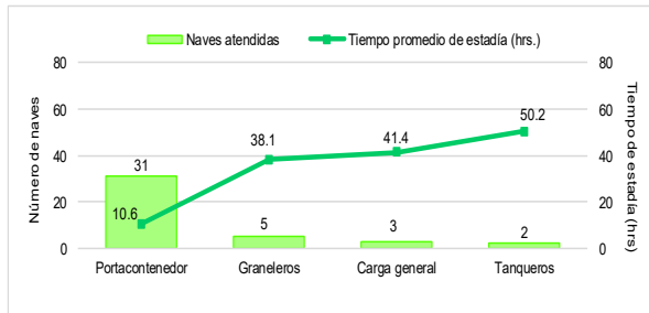
Gráfico N°1 Tiempo promedio de estadía de los amarraderos por tipo de naves en el TP Paíta - TPE, Julio 2021
