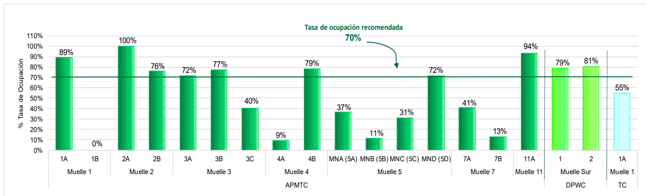
Gráfico N°10 Tasa de ocupación de los muelles de los terminales portuarios del Callao administrados por APMTC, DPWC y TCSA, julio 2021
