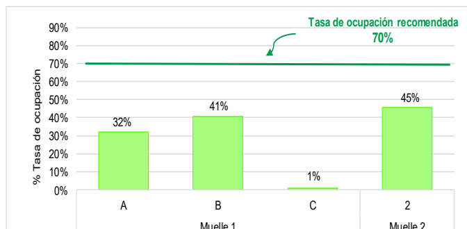
Gráfico N°6 Tasa de ocupación de los amarraderos de TP Paita -TPE Julio 2021
