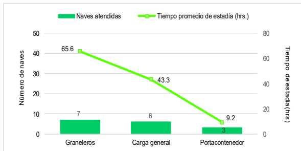
Gráfico N°3 Tiempo promedio de estadía de los amarraderos por tipo de nave en el TP General San Martín - TPP, Julio 2021
