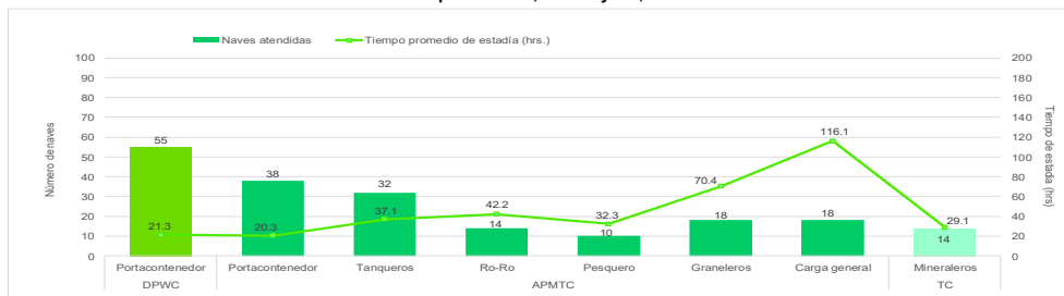
Gráfico N°5 Tiempo promedio de estadía de las naves según tipo, en los amarraderos de los terminales portuarios del Callao administrados por APMTC, DPWC y TC, Julio 2021
