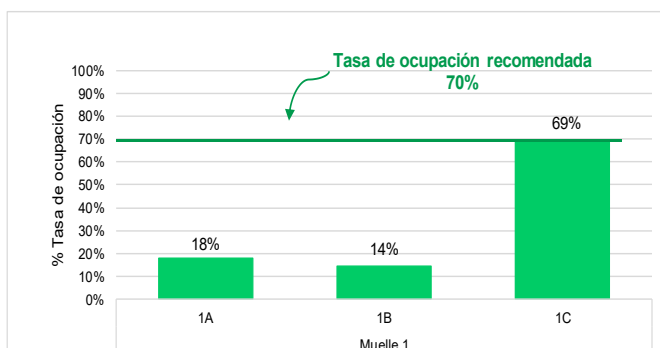
Gráfico N°7 Tasa de ocupación de los muelles del TP General San Martín - TPP Julio 2021
